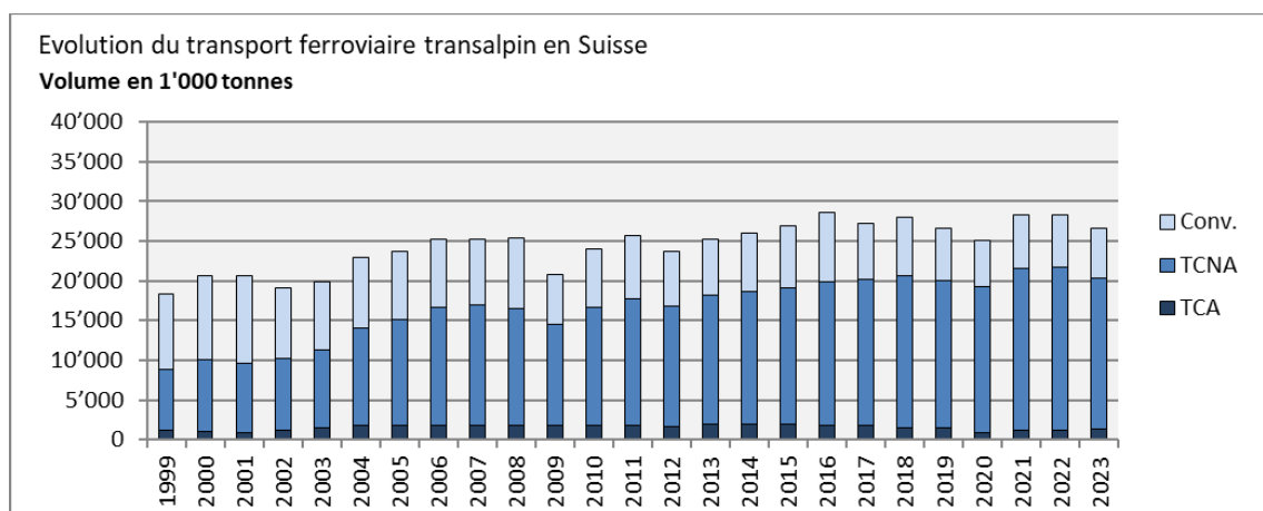
Figure 15: Evolution du transport ferroviaire transalpin en Suisse ; en milliers tonnes nettes
