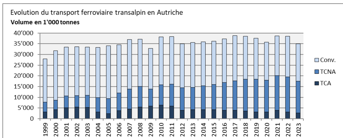
Figure 16: Evolution du transport ferroviaire transalpin en Autriche ; en milliers de tonnes nettes
