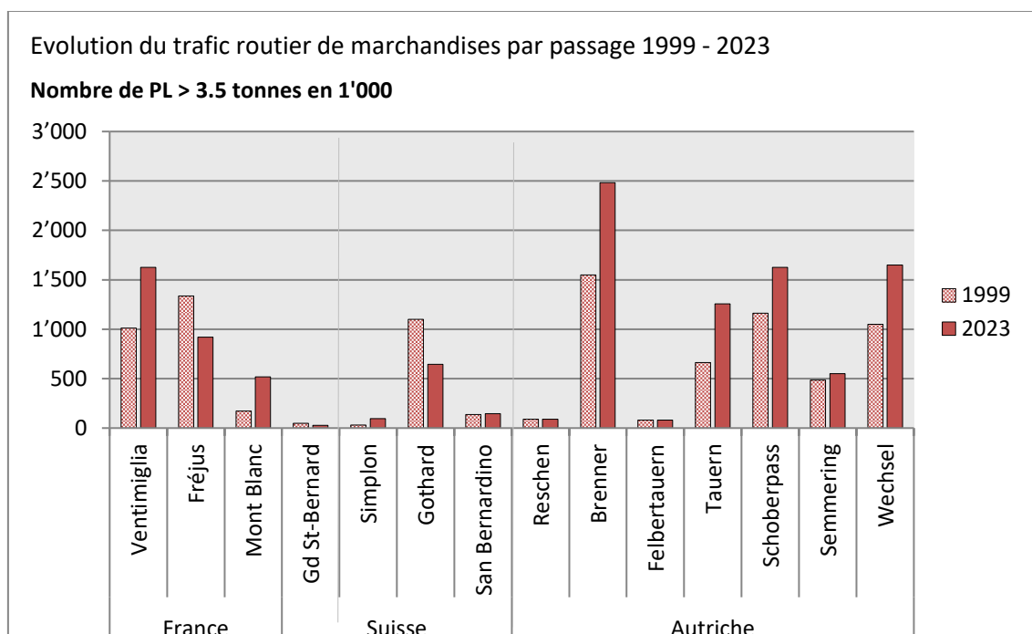
Figure 13: Evolution du trafic routier par passage 1999 - 2023
