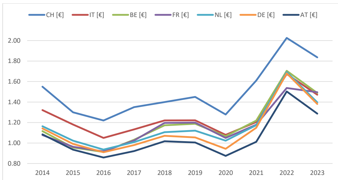
Figure 32: Evolution des prix du diesel depuis 2014
