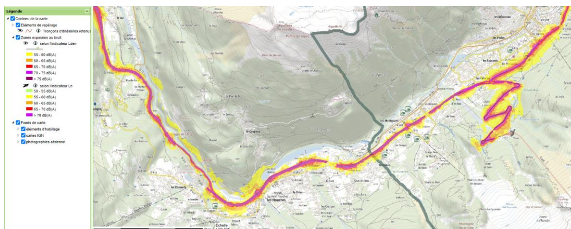
Figure 47: Emissions sonores le long de la RN 205, à la hauteur de Chamonix et de l'accès au tunnel du Mont-Blanc (indicateur L_{den} ) – Source : Géo-IDE carto, Carte des zones exposées au bruit, 2021
